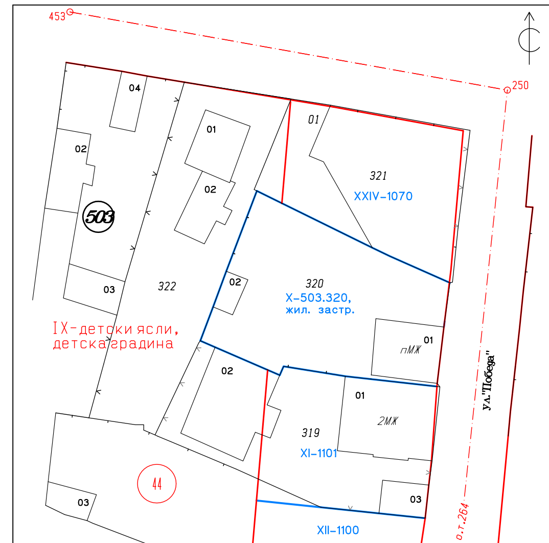
Плана за регулация за нови УПИ IX-детски ясли, детска градина, УПИ XXIV-1070, УПИ XI-1101 и УПИ X-503.320, жил. застр. от кв. 44 по имотни граници на ПИ 39921.503.320 по КК.
