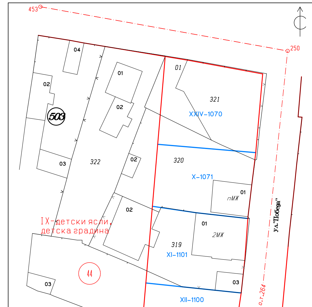
Комбинирано извлечение от действащ регулационен план, за част от кв. 44 по плана гр. Крчим, общ. Крчим, одобрен със Зап. № 902/1982г., с имотни граници по действаща кадастрална карта на гр. Крчим.
