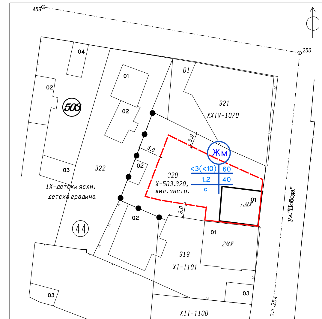
Плана за Застрояване за нов УПИ X-503.320, жил. застр. от кв. 44 по плана на гр. Крчим.
