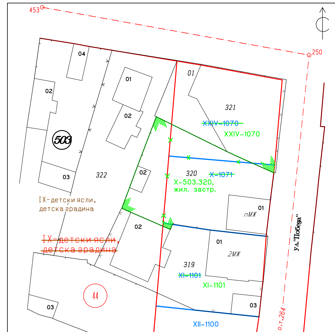
Изменение на плана за регулация за УПИ IX-детски ясли, детска градина, УПИ X-1071, УПИ XXIV-1070 и УПИ XI-1101, кв. 44 по плана на гр. Крчим, като се образуват нови УПИ по имотни граници на ПИ 39921.503.320 по КК.
